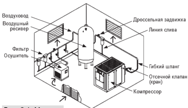
Рис. 2.1: Монтаж
