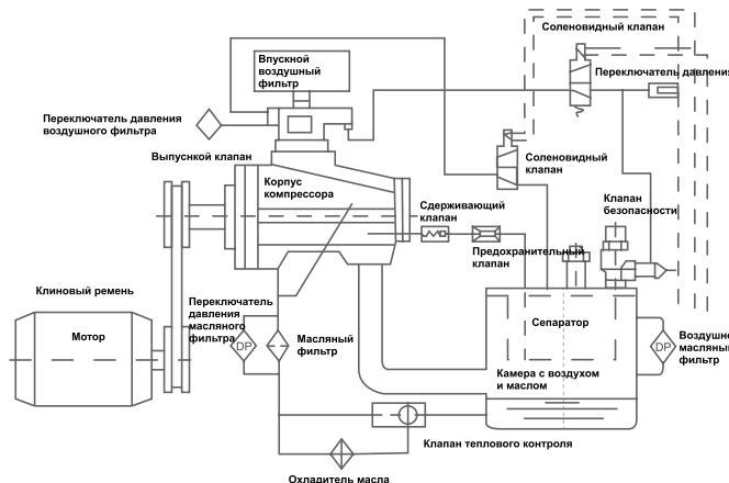
Схема технологического процесса (30 кВт)
