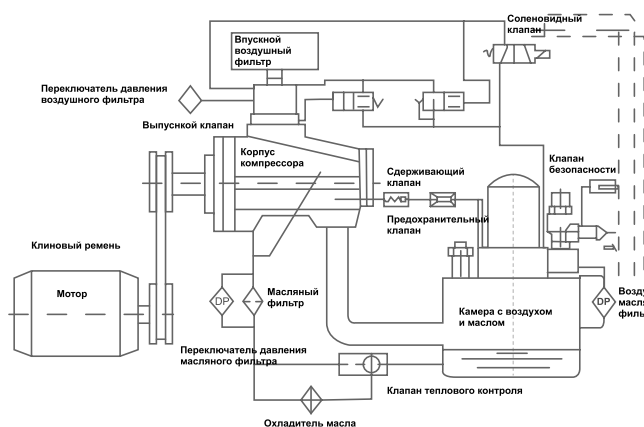
Схема технологического процесса (22 кВт и ниже)
