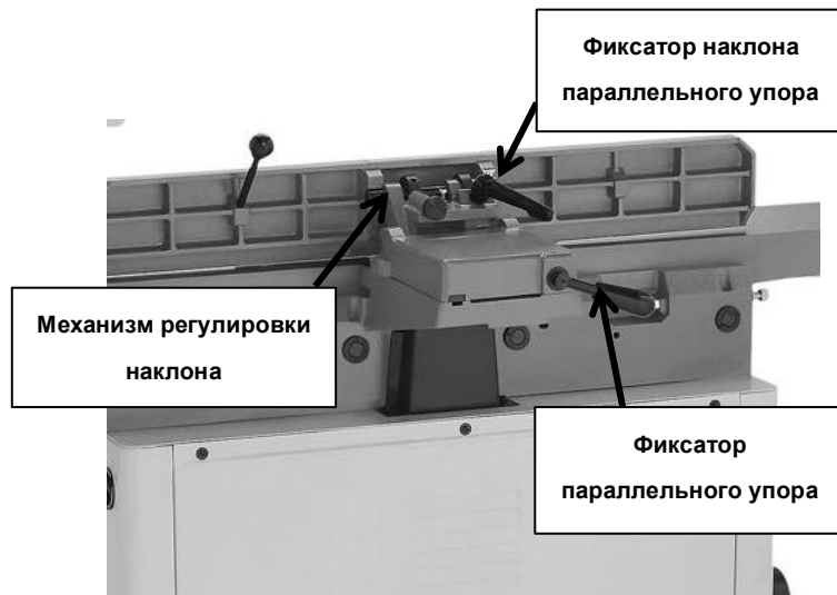
Рис.3 Расположение ручек фиксации параллельного упора.
