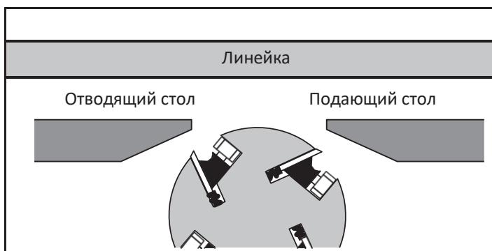
55. Отводящий и подающий столы установлены правильно.
