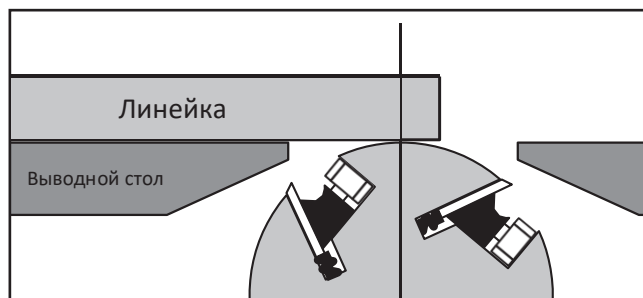
Рисунок 48. Регулировка выводного стола
