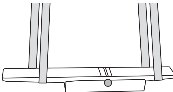
Рис. 12 Использование подъемных ремней для подъема фуговального узла
