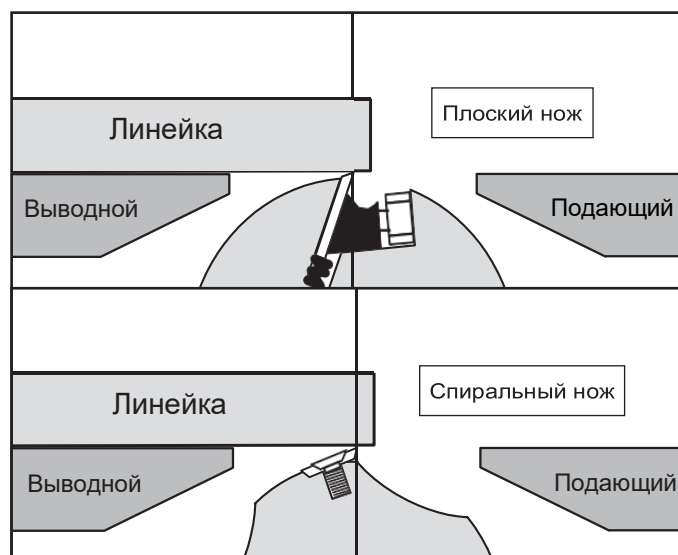
Рис. 24 Используйте линейку для проверки высоты стола подачи.
