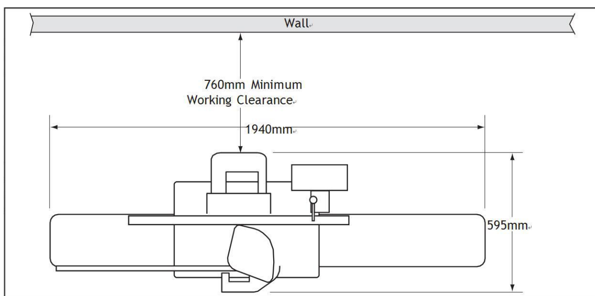
Рисунок 8. Минимальные рабочие зазоры.
