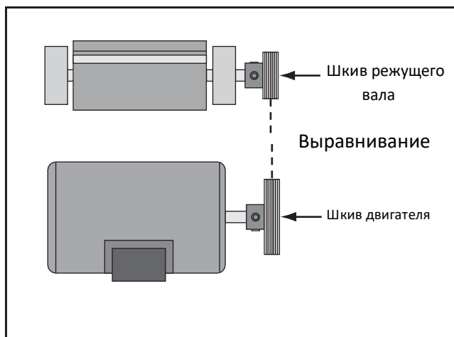
Рис. 42 Выравнивание шкивов
