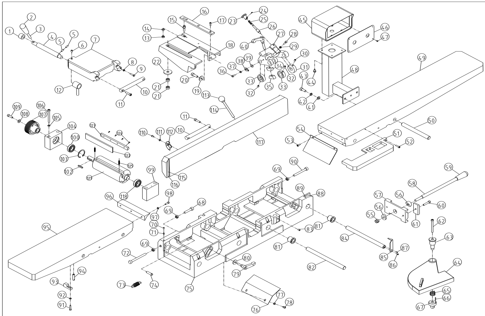
Чертеж №1 Общая схема
