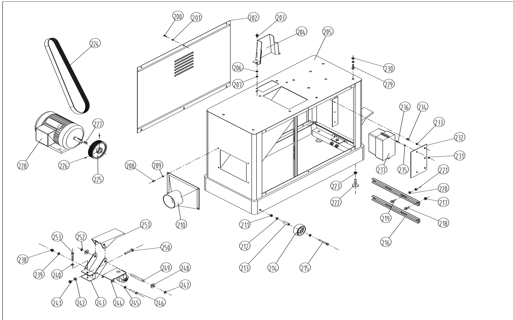
Чертёж №2 Корпус
