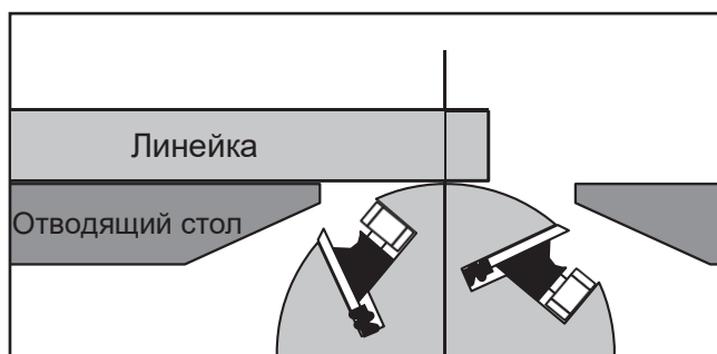
Рис. 52 Регулировка отводящего стола.
