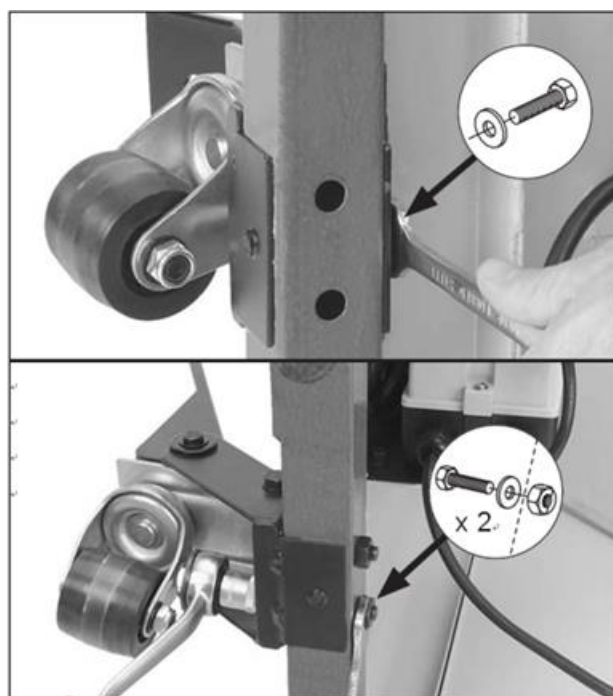
Рис. 10 Установка педали.
