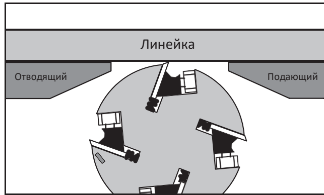
Рис. 61 Подающий стол даже с выпускным столом.
