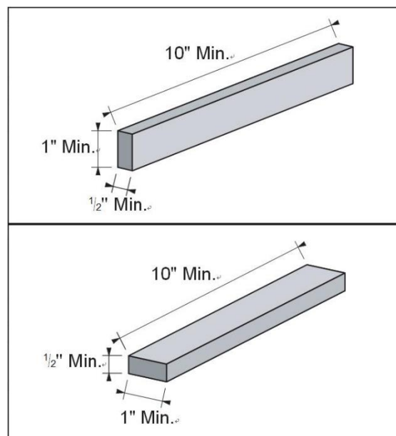
Рис. 30 Минимальные размеры заготовки.
