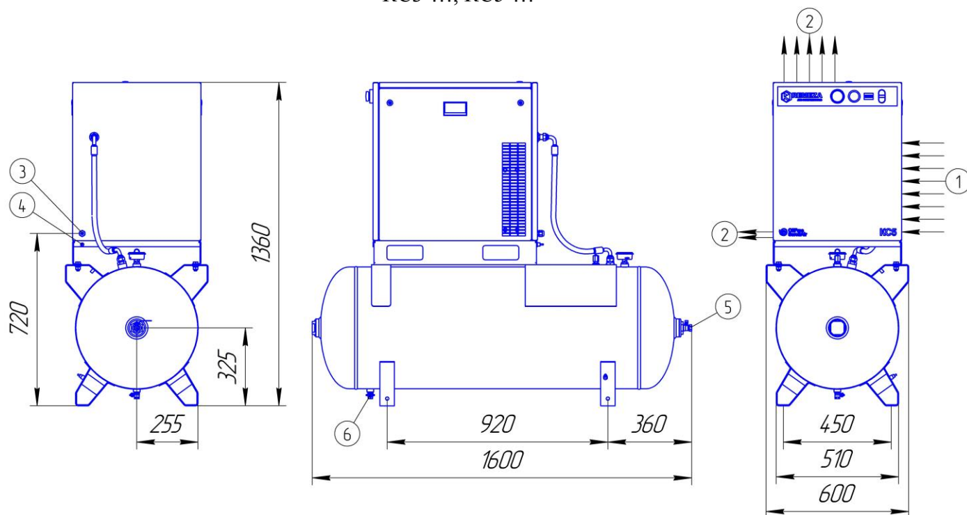
Рисунок А1 – Присоединительные и установочные размеры компрессорной установки KC3-..., KC5-...
