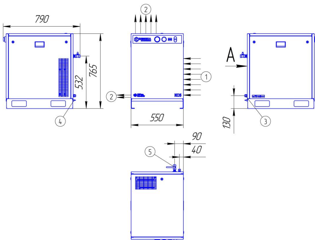
Рисунок А1 – Присоединительные и установочные размеры компрессорной установки KC3-..., KC5-...
