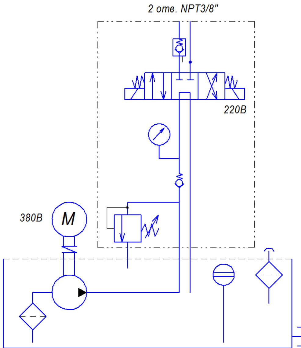
Рис.2 (Гидравлическая схема)
