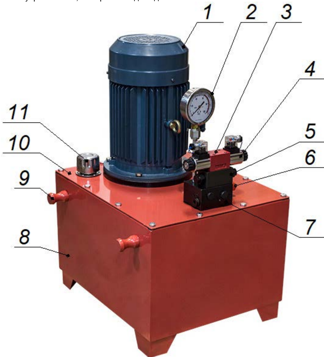
Рис.1 (Устройство маслостанции)
