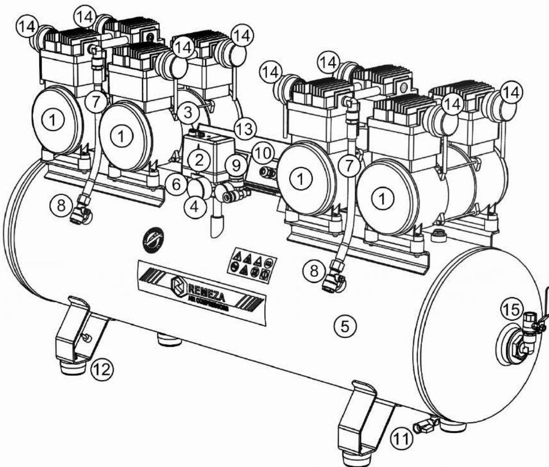
Рисунок 5 - Общий вид компрессора СБ4-150.OLD20x4
