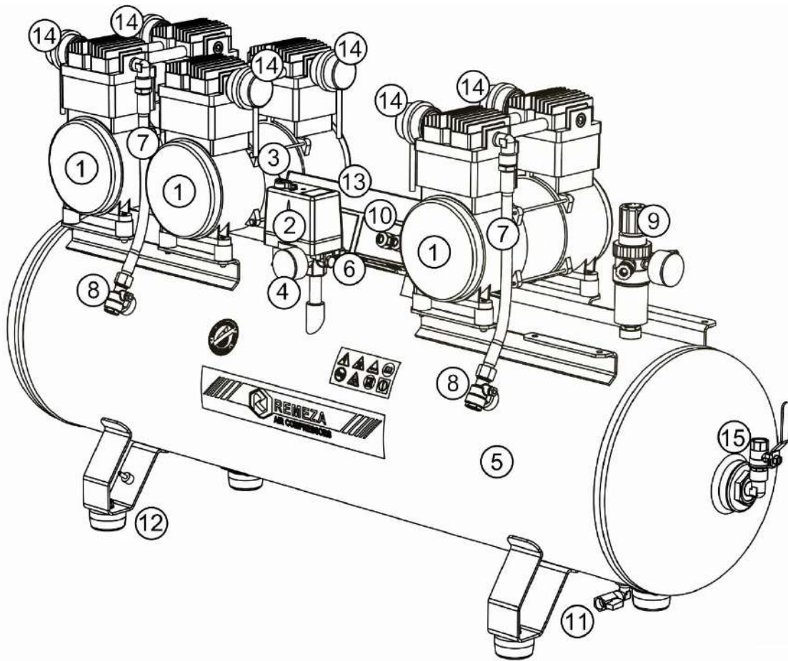
Рисунок 4 - Общий вид компрессора СБ4-150.OLD20x3
